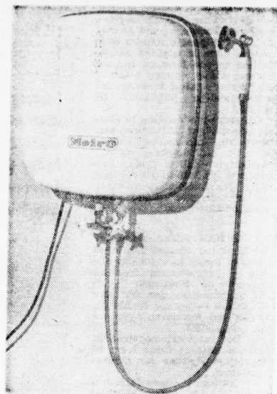
15 liter el-vandvarmer. Vandvarmeren er hvidemaljeret, og udvendig måler den 60×51×21 cm. Det indstillige temperatur- område er fra ca. 30 gr. til ca. 70 gr. C.
