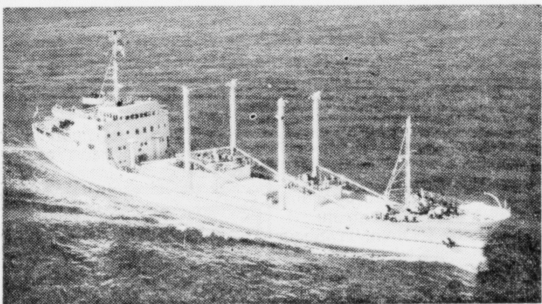
Eimskipafelagið hevur gjørt keypsáttmála um frystiskipið »Echo» smíðað í Hollandi í 1961. Ms. »Echo» tekur 1400 tons av frystum fiski, tað er 2120 tons stórt. Ferðin er 14—14,5 mil.
