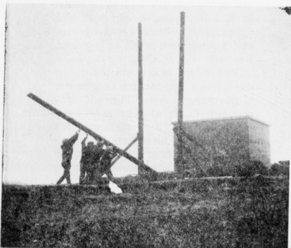
Endursendingarstoðin á Støðlafjalli: antennumastrar verða reistar
