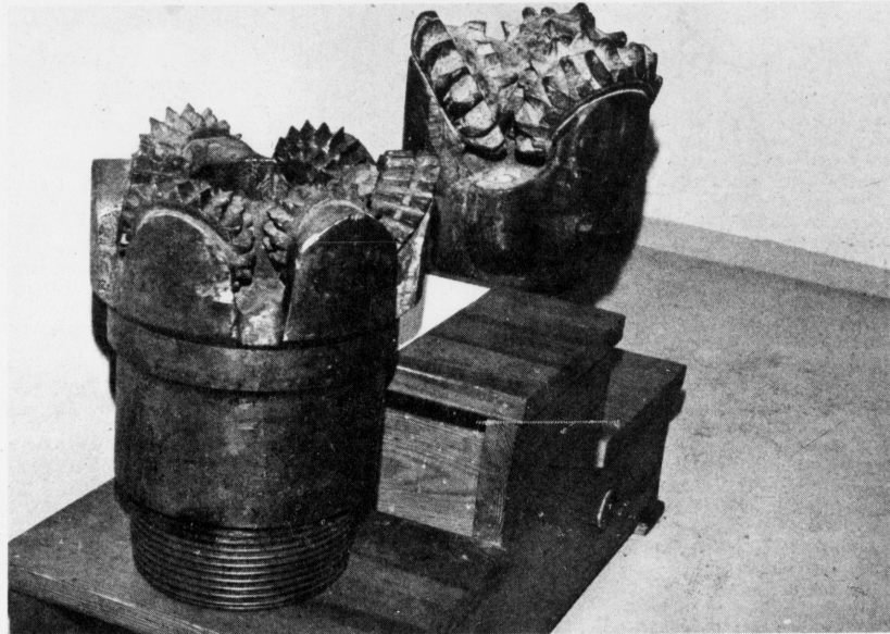
Borikrúnur ið nýttar vóru til royndarboringar á Danfæltinum.
