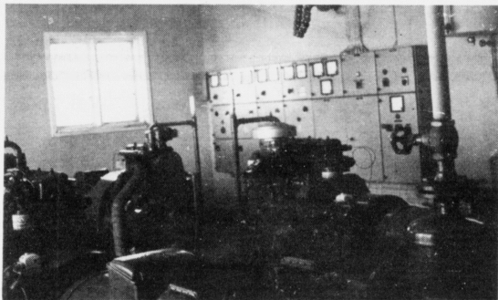
Vitastøðin á Borðuni er útgjörd við 4 ljósmotorum. Herav eru tveir útgjördir við kompressara til tokulúðurin á Borðtanga
