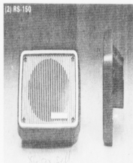
Modell RS 150 pr. stk. 43,00 kr. 10 W frittstandandi ella til innbygging
