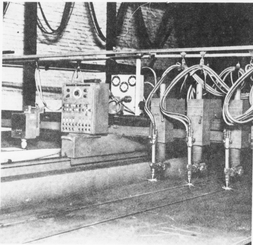
Nýggi skreibrennarin hjá Skála Skipasmiðju
