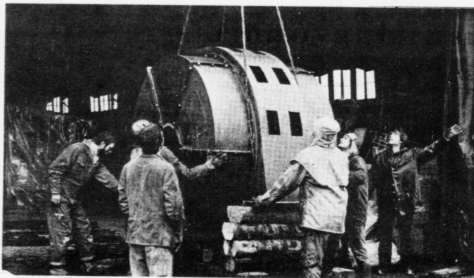
El-generatorurin vigar 12 tons. Hann er keyptur úr Svøríki
