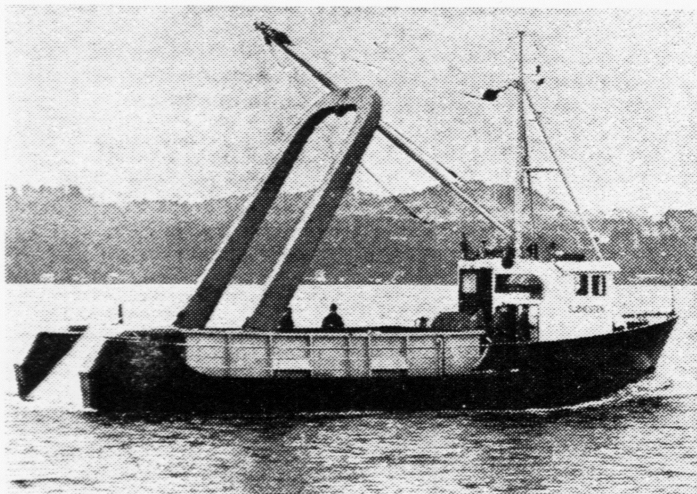
Norðmenn hava eisini gjørt bátar til einans at trola eftir tara. Hesin báturin er 57 føtur langur, hevur ein 180 HK dieselmáskinu og og siglir 9 mil
