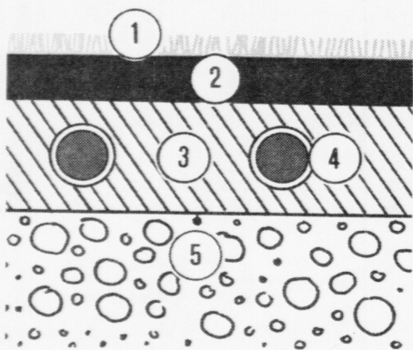
Poligrasvøllurin: 1. poligras, 2. gummibelegningur, 3. asfalt, 4. møgulig hitarørir í vøllinum og 5. steinsetingin.
