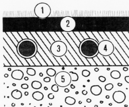
Poligrasvøllurin: 1. poligras, 2. gummibelegningur, 3. asfalt, 4. møgulig hitarar í vøllum og 5. steinsetingin.
