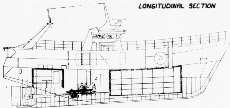
Soleiðis sær hann út. Tær 850 hestakreftirnar og skrávudysan geva bátinum 13 mila ferð
