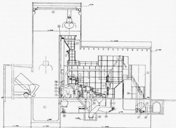
Skitsa av brennistøð. Rusk, mold og glas og annað burturkast verður koyrt beinleiðis í grøvina. Hetta verður tikið upp av grabbara og koyrt ígjøgnum anleggjið. Ein maður stýrir øllum arbeidinum á einum sjónvarpskermi
