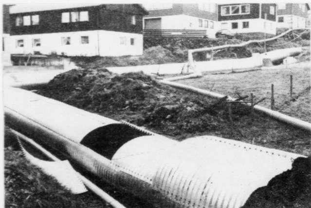
Stálið í rørnum er 3,4 mm. Botnurin verður styrktur við einum betonglag. Vinstrumegin sæst onnur kloakkleiðingin. Høgrumegin eru rørin, sum áin er beind í, meðan arbeiði verður
