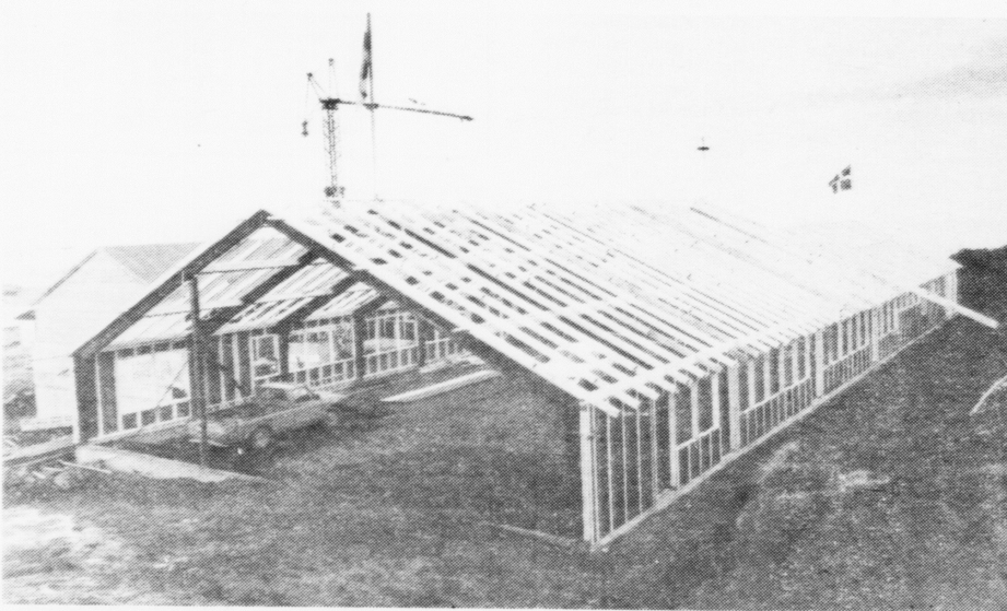
Verkstaðurin Vón á Argjum. Í kjallaranum í ti niðara partinum verður parkeringspláss. Næmingaheimið hjá Skúlanum á Trøðni skal byggjast omanfyri verkstaðin. Myndin er tikin mikudagin, tá reisigildið var
