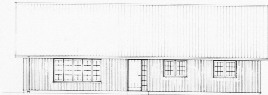
FAÇADE MED NOVVEDUP. MÅL: 1:50
