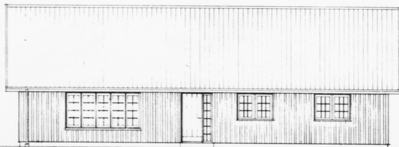
FACADE MÍÐ HÖVUDENDI. MÁL. 1:150
