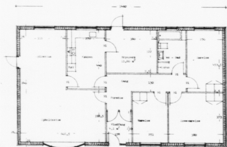
TAFEL. MÁL. 1:150 HÚSISAMMANTÁL 113 m 2 . OPPL. 113 m 2 . OPPL. 113 m 2 .
