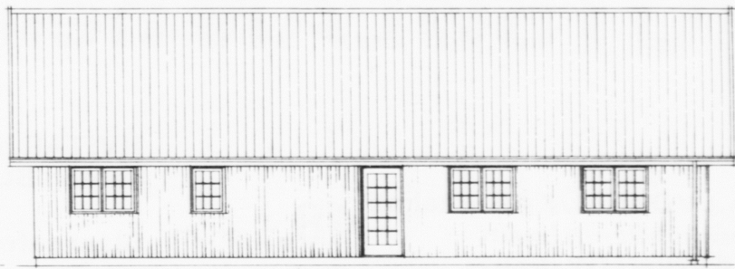
FACADE MED HRYGGSDØR.
