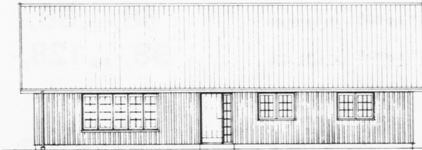
FACADE MED HOVEDDØR. MÅL. 1:50
