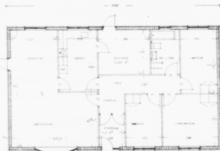
PLAN MÅL: 1:50 ISODAN HÚSIÐ 1984
