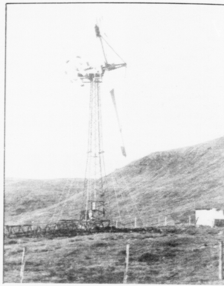
Vindmyllan hjá Birgiri og Helga Enni uppi á innara Hváli á Tvøroyri. Myllan hevur koyrt síðani í juni
