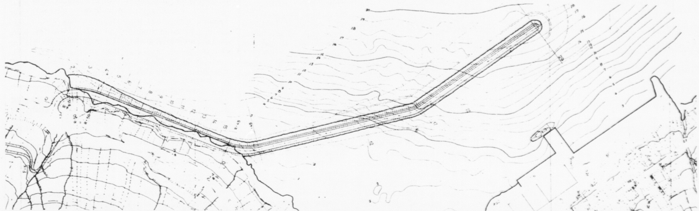
Eitt 300 metra langt grótkast fer at gera havnina kyrra. Grótbrotið á Víkanesi sæst uttast til vinstru
