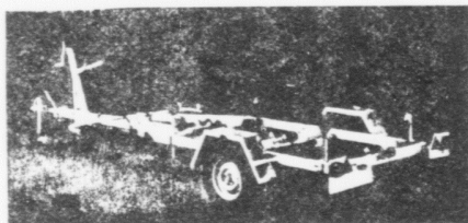
Type VA 800 B
