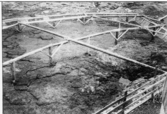
Køsturin, sum er grivin niður á hellu og hevur timburbygging, tekur 750 kubikmetrar. Ætlingin er at stoyppa ein kant framvið. Hann er gjørður soleiðis, at tak kann leggjast á. Har hann er djúpast er hann trýggjar metrar. Tøðini verða pumpað á bœin gjøgnum rør. Pumpan situr á traktorinum. Kostnaðurin liggur um 70.000 kr.
