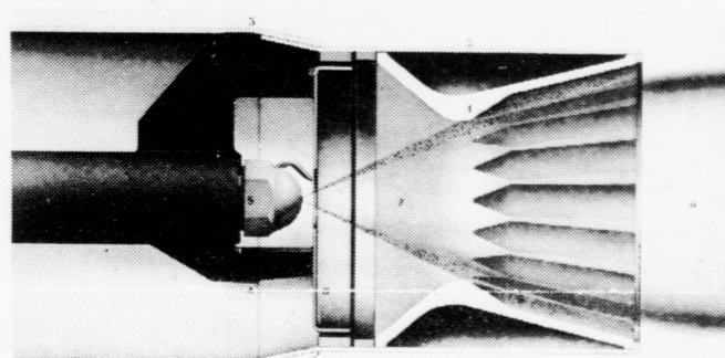
Tværsnit af brænderen i det nye oliefyr-system. Det keramiske fordampenhoved til højre for dysen opfanger de »tunge« oliedråber, som bringes til fordampning og forbrænding, hvorved indholdet af uforbrændt olie i skorstenstrøgen reduceres til et minimum. Tallene på snitbilledet har følgende betydning: 1. fordampenhoved, 2. holder, 3. brænder, 4. blandeskiveholder, 5. oliefyde, 6. blandeskive, 7. flammekegle, 8. forstørrelseskegle, 9. flamme.
