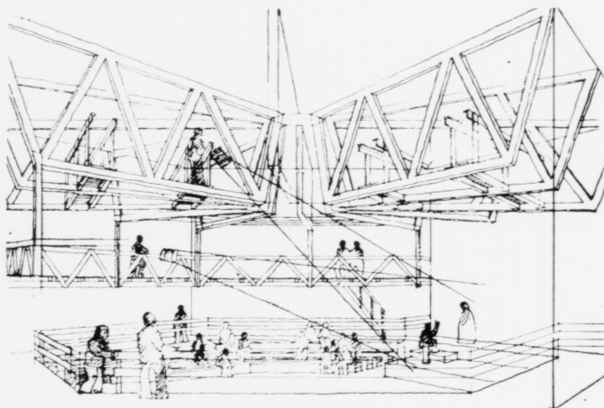
Herning arena-teater. En 6-kantet sal, som er forberedt til også at kunne rumme prosceniums-teater, idet den ene væg omdannes til sceneåbning. (Arkitekterne Tyge Arntfred og Viggo Møller-Jensen).
