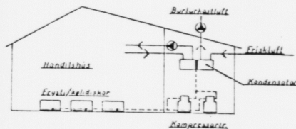
Mynd 13. Kólianlegg nýtt sum hitapumpa í handilshúsi.
