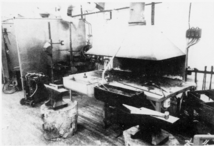
Teir sleppa eisini at royna, hvussu tað er at smíða, meðan jarnið er heitt. Vinstrumegin á myndini sæst eitt av sveisingarrúmunum
