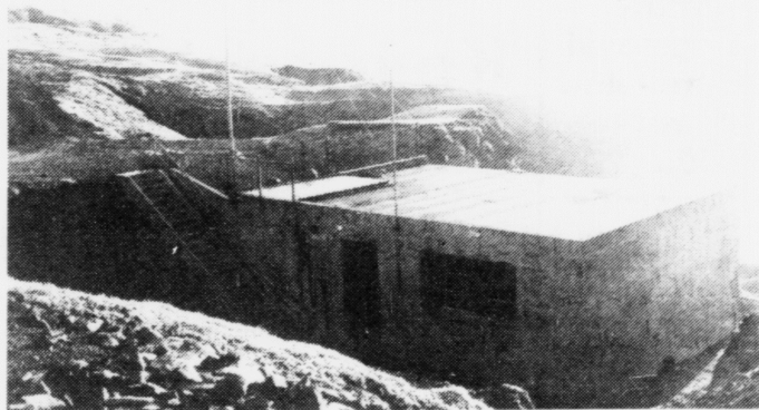
Vatnverkið í Botni á vestur síðuni á Suðuroynni. Hetta er tað elsta el-verkið í Føroyum. Húsið við turbinunum stendur heilt niðri við sjóvarmálan. Vatnið kemur úr rørum úr Ryskivatni og Miðvatni oman fyri born og gjøgnum tunnel úr Vatnsnesi við Hov
