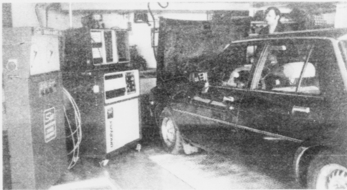
Ein bilur í tí nýggja rullu-royndar-tólinum hjá Sjúrða Strøm í Vági. Uttast panelið at stilla rullu-royndar-tólið inn á. Síðan sjálvur motor-testarin
