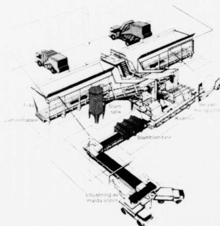
Útbúnaður við tveimum kvørnum
