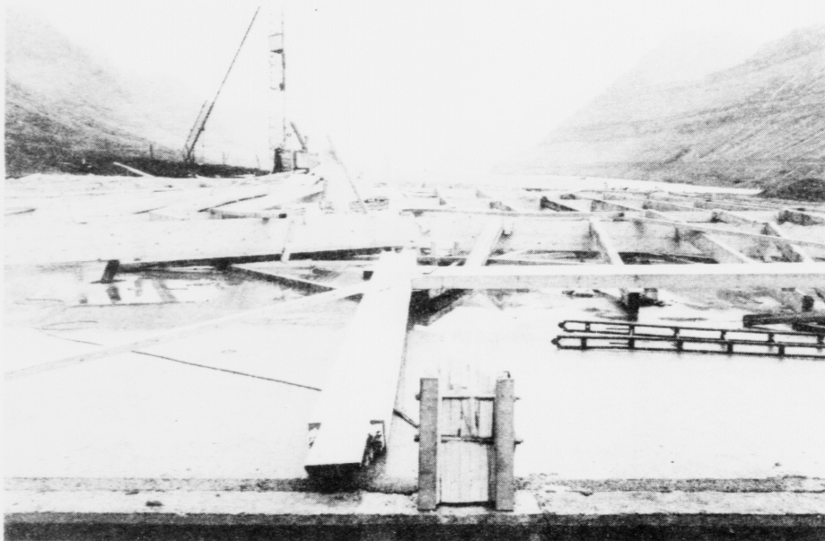
Henda myndin varð tikin, tá skúlin í Hvannasundi herfyri rapaði av vindi. Av tí at tað er sera vindhart á ókinum, har skúlin stendur, hevur bygðaráðið í Hvannasundi samtykt, at stoypa skúlan upp aftur í betong
