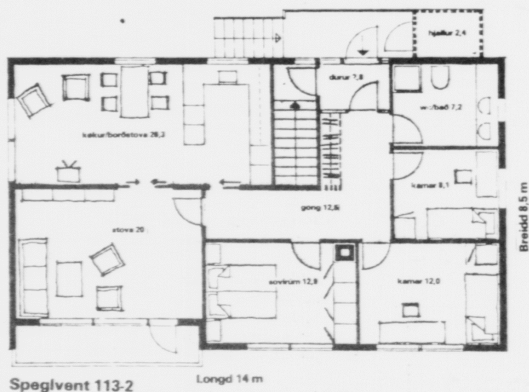
Speglivent 113-2
