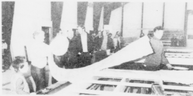
Stórviðurin í elementinum er komin upp á pláss og uttasta lagið av glasull, 5 cm, verður lagt í
