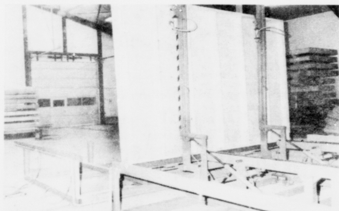
Eitt element verður vent við. Tveir armar færa elementíð runt. Hond verður bert nýtt til eitt fjarstýrt tól
