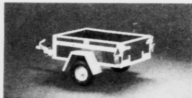
VARIANT PÁHÆNGSVOGN Type VA 300-2-122 Totalvægt: 300 kg Nyttelast 225 kg Ladmál 122 x 85 x 35 Hjúlstørrelse 400 x 8
