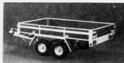
VARIANT PÁHÆNGSVOGN Type VA 750-244 Totalvægt 750 kg Nyttelast 525 kg Ladmál 244 x 150 x 30 Hjúlstørrelse 145 x 10
