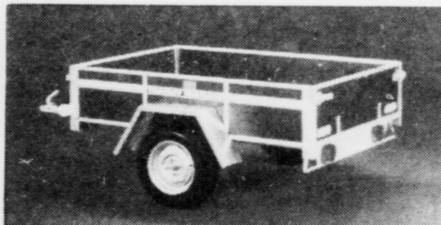
VARIANT PÁHÆNGSVOGN Type VA 501-190 Totalvægt 500 kg Nyttelast 350 kg Ladmál 190 x 122 x 40 Hjúlstørrelse 155 x 13
