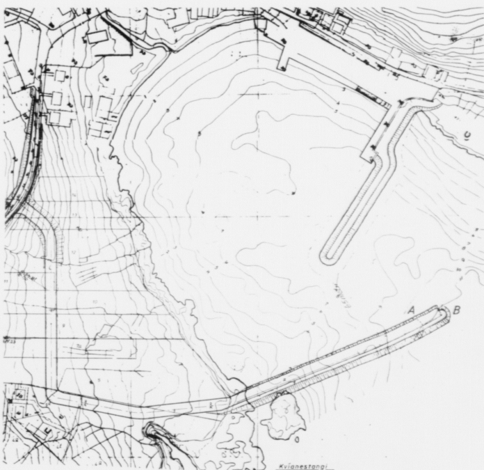
Uppskot til ætlaða grótkastið. A og B eru møguleikarnir. Tekning frá Landsverkfæðinginum.
