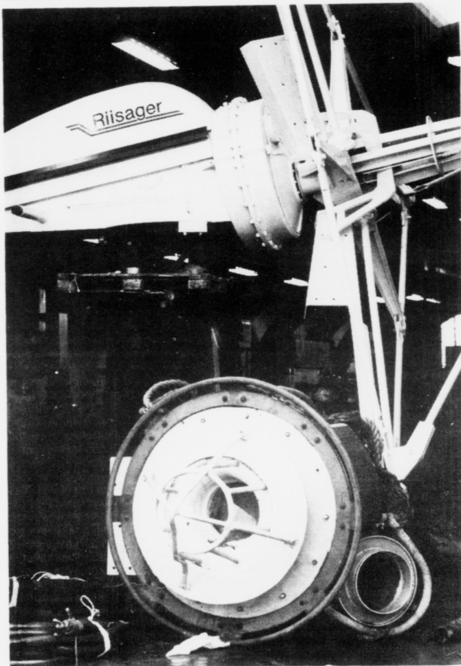
Partur av vindmyllu, sum verður gjørd á verkstaðnum hjá J. K. Joensen í Miðvági. Fremst á myndini pumpan hjá Sólbjørn Jacobsen, telefonverksstjóra, ið skal nýtast umborð á svartkjaftaskipum
