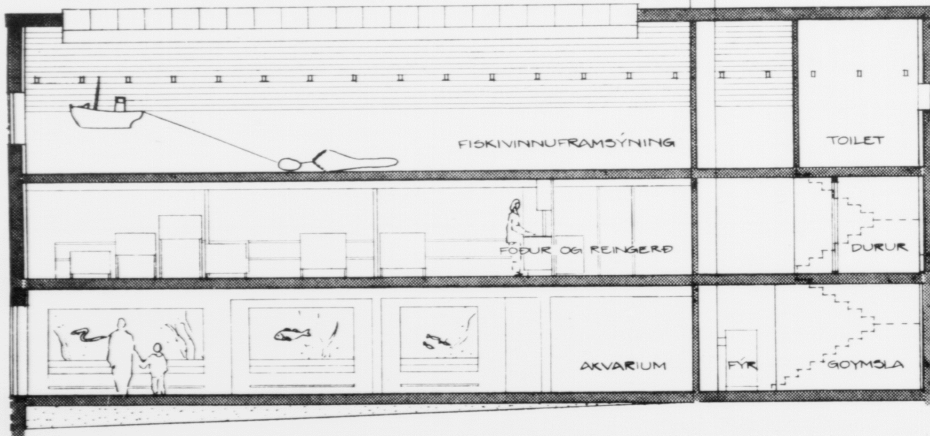
Longdarskurður - mál 1:100.
