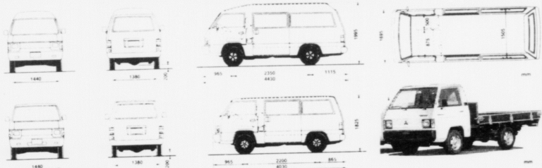
LONGBODY PANEL VAN
