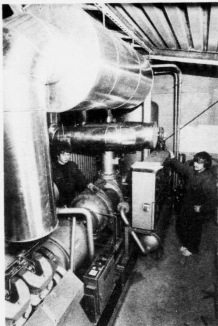
Á ísvirkinum hjá Bacalao hava teir nú í eina tíð brúkt egnan dieselmotor til ísframleiðsluna istaðin fyri at keypa streym frá SEV
