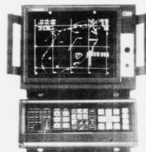
Informationerne præsenteres på radarens 14" dagslysskærm i 7 forskellige farver. 3 kortudsnit (hukommelsesblokke) med til sammen 1.500 plotdata. Samtidig visning af videoplot og radarbillede. 4 forskellige billedfremstillinger.
