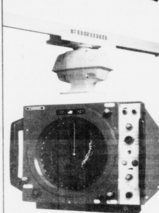
Model FR-1011 1/4-1/2-3/4-1 1/2-3-6-12- 24-48-72 sømil 10 kW sendereffekt 10" PPI/16" linse 4' eller 6 1/2' antenne Var. afstandsmåler std.
