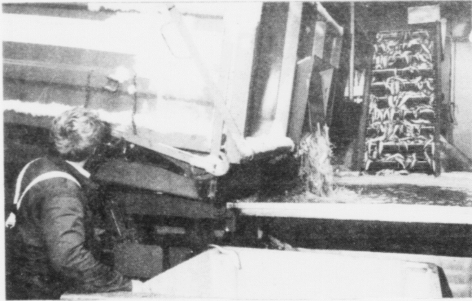
Konteinari við 15 tonsum av svartkjafti verður koyrdur inn á virkið, har svartkjafturin fer í eitt stórt kar við vatni, og síðani fer hann inn á flutningsbandið og viðari til flakamaskinurnar
