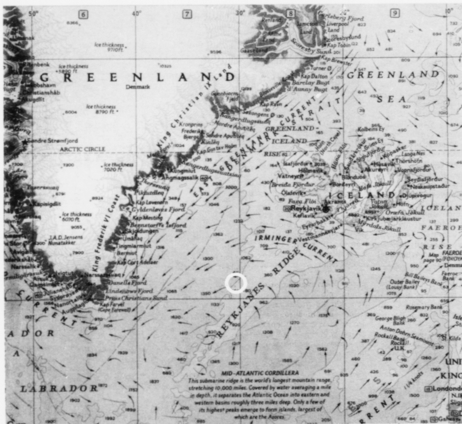
Sirkulinn sýnir, hvar íslendingar raktu við kongafisk í 1982 og 83. Russar fiskaðu 60.000 t. á Reykjanesrygginn eitt árið.
