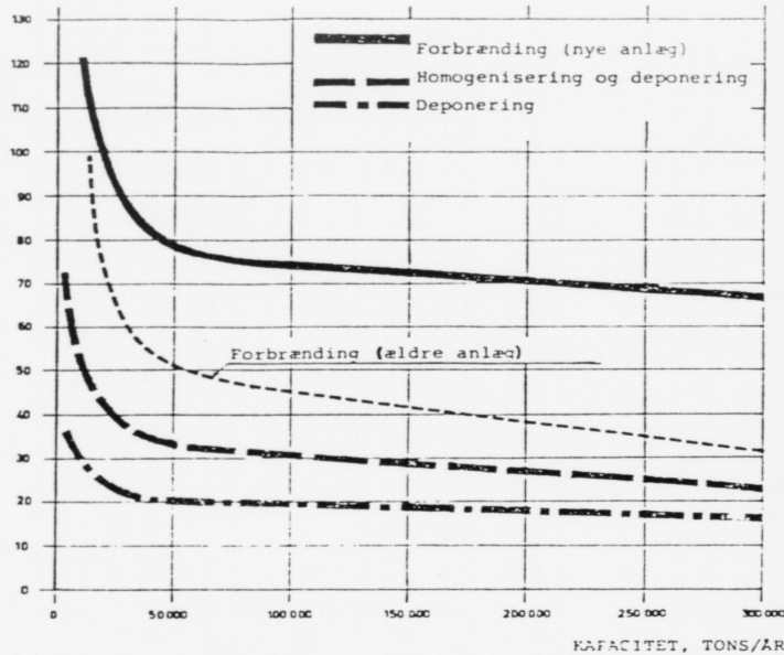
Fig. 4.5. Behandlingsudgifter (sv.kr./ton) som funktion af anlæggets størrelse (tons/år). Priseniveau 1973. (K-KONSULT).
