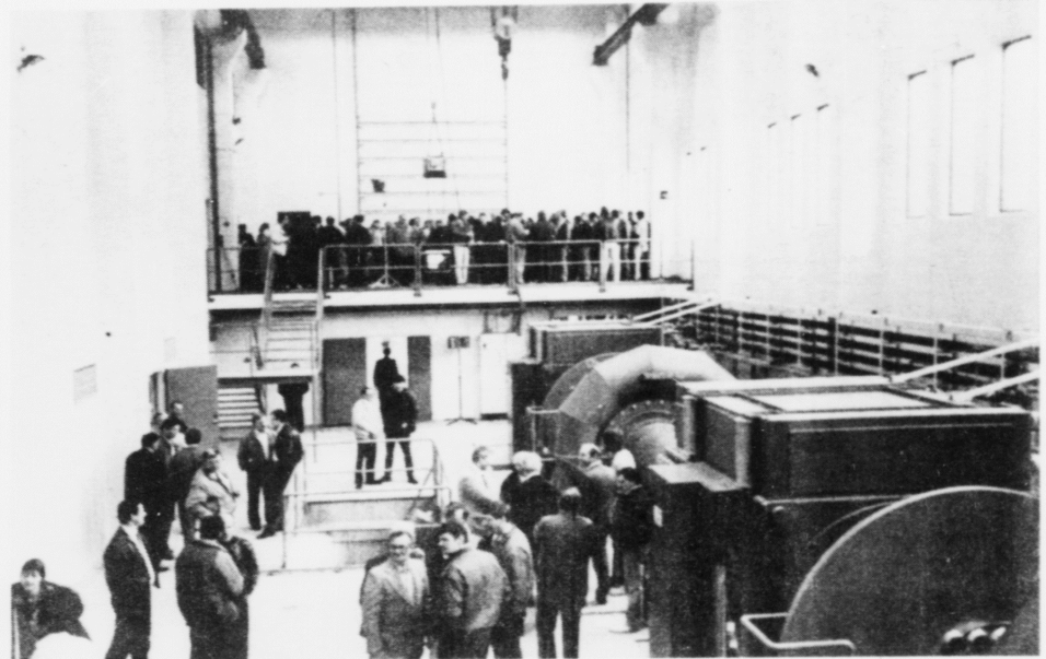
Inni á Eiðisverkinum. Her standa báðar turbinurnar, sum, tá Eiðisverkið er fult útbýgt og hevur fingið nógv mikið av vatni, kann framleiða 60 mió. kWt. Hetta er tað sama sum øll hini vatnorkuverkini hjá SEV gera í dag
