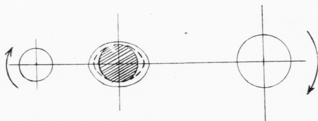
Mynd 6. Nú eru góðir 7 dagar lidnir síðan fyrra kvarter. Nú er fullmáni, flóðaldurnar virka nú aftur sama veg, og um 1 - 2 dagar er aftur harðasti streymur.
