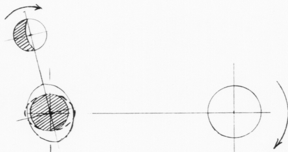
Mynd 5. Enn eitt umfar, mánin veksur, og streymurin harðnar.
