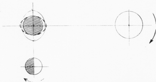
Mynd 7. Umleið 7 dagar aftaná fullmána hava vit seinna kvarter. Flóðaldurnar virka nú aftur hvør sín veg, t.v.s. tann samlaða flóðaldan hevur nú aftur sitt minsta virði, og vit hava fyri aðru ferð besta streym um 1 - 2 dagar.
