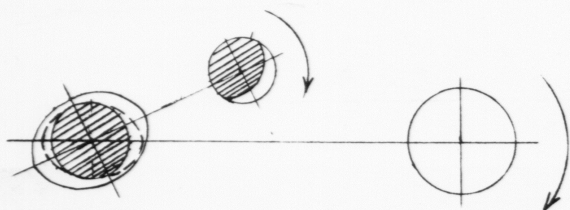
Mynd 3. Enn eitt samdøgur er liðið, og sólin er komin enn eina ferð runt jørðina. Máin er nú í síni ferð runt jørðina seinkaður umleið hálvan annan tíma í mun til sólina — streymurin linkar.
