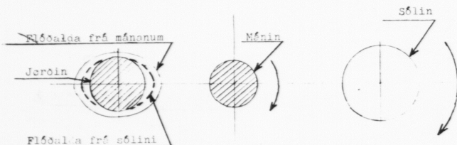
Mynd 1 — Byrjunarstöða. Niða, ella tendring (Máin er myrkur). Flóðaldurnar báðar virka sama veg. 1 - 2 dagar aftaná er harðasti streymur.
