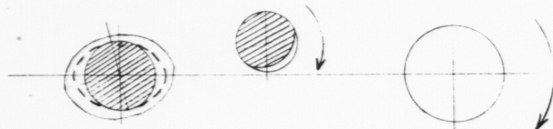
Mynd 2. Eftir einum samdøgurði er sólin nú komin eina ferð runt jørðina. Máin er tó ikki komin runt enn, tí hann hevur umleið trý korter longur um ferðina. Sum myndin visir, virka flóðaldurnar nú ikki sama veg — streymurin linkar.
