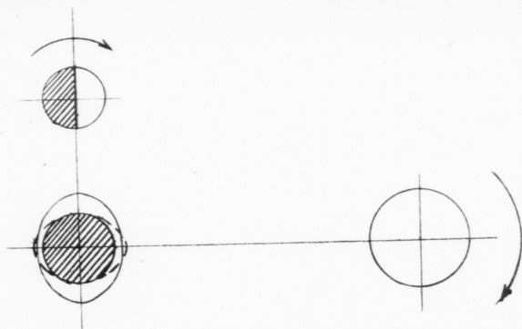
Mynd 4. Nú leypa vit fram til 7. samdøgur. Máin er nú seinkaður fjórðings umfar í mun til sólina. Nú er fyrra kvarter — máin er hálvur. Atdráttarmegin hjá mánanum og sólina virka nú soleiðis, at tann samlaða flóðaldan hevur sitt minsta virði. 1 - 2 dagar aftaná er besti streymur.
