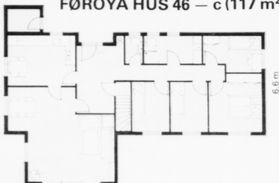
FØROYA HÚS 46 — c (117 m 2 )
