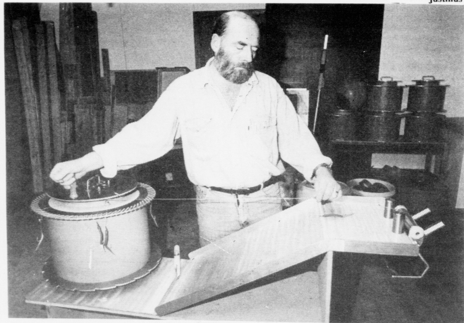
Óg her er endaliga úrslitið. Nýggja snurran er 50 sentimetrar í diametrar og kostar 12.000 krónur. Hon kann nýtast til nylonlínu upp til 200 húkar og 70 húkar á toskadorg. Mynd Kalmar
