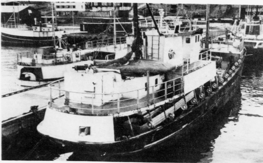
Nógv føroysk skip eru útgjørd við Vágasnellum. Her er tað eitt fiskiskip í Klaksvík, sum hevur ikki minni enn 14 av teimum teldustýrdu snellunum frá Oilwind. Mynd jan
