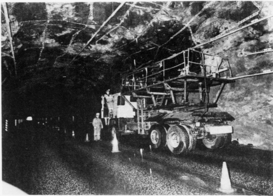
Net verður spent uppundir, so grót ikki dettur niður, og plátur seta teir uppundir, har tað lekur.
